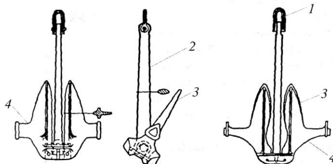
Рис. 9-4. Якорь Матросова:
